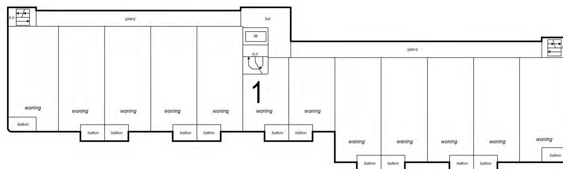
3e Verdieping 1:200
