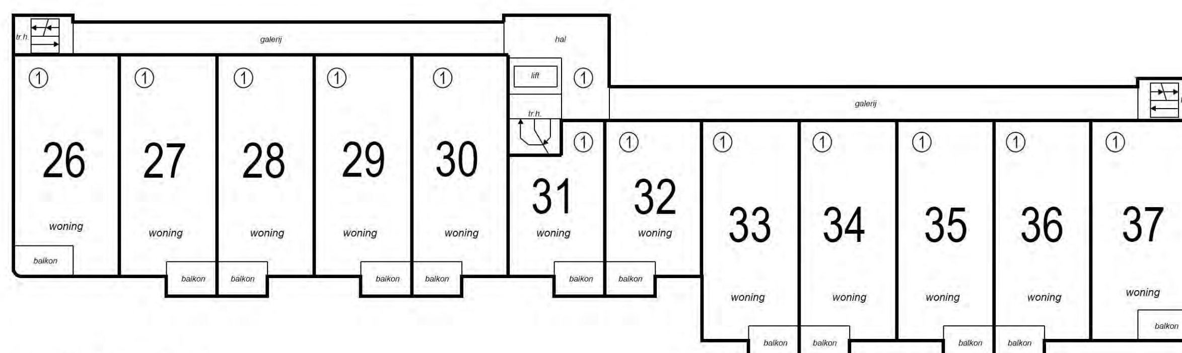
2e Verdieping 1:200
